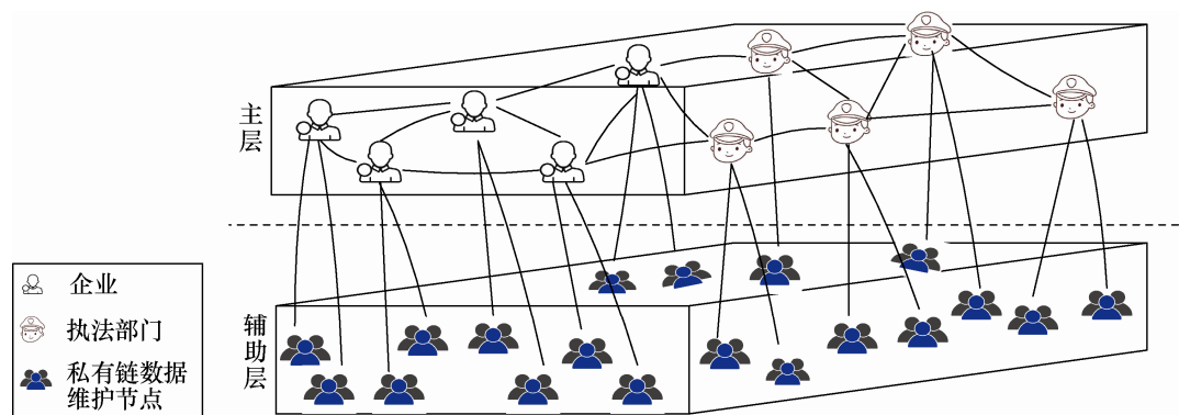
图1 双层架构体系
