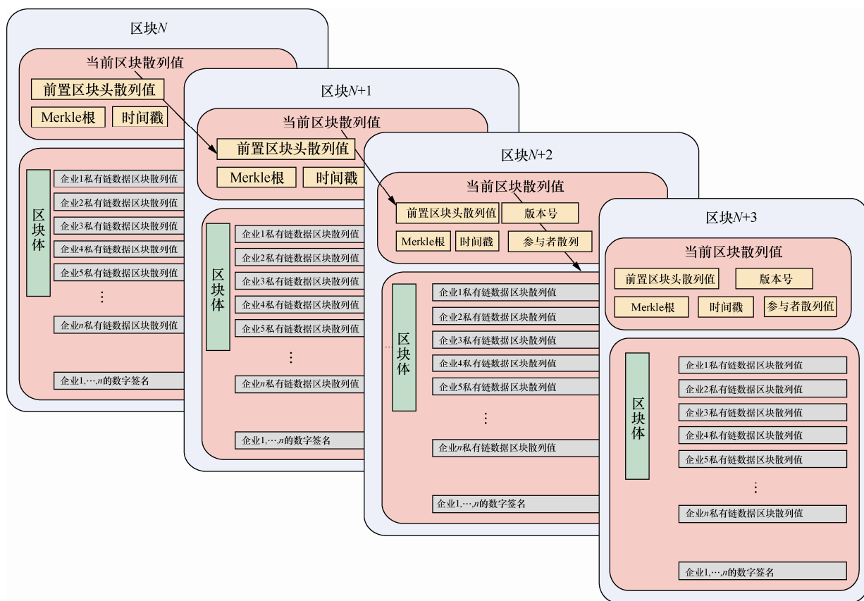
图3 主层联盟链的数据结构
