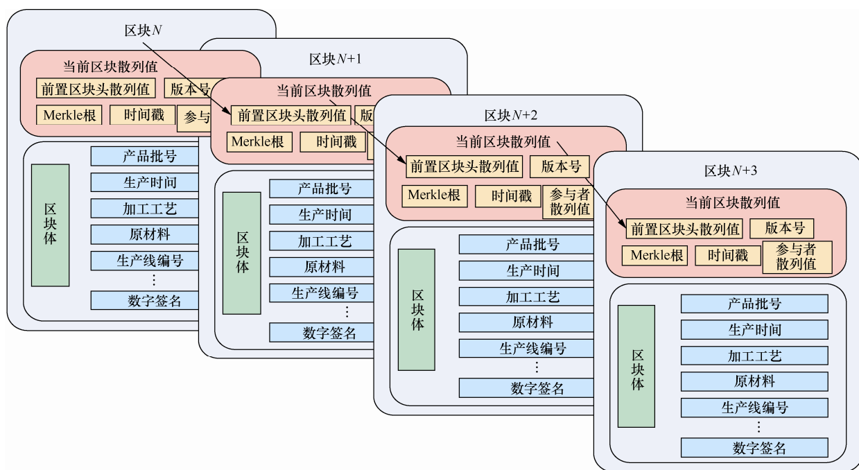
图2 生产企业私有链数据区块结构的示例
